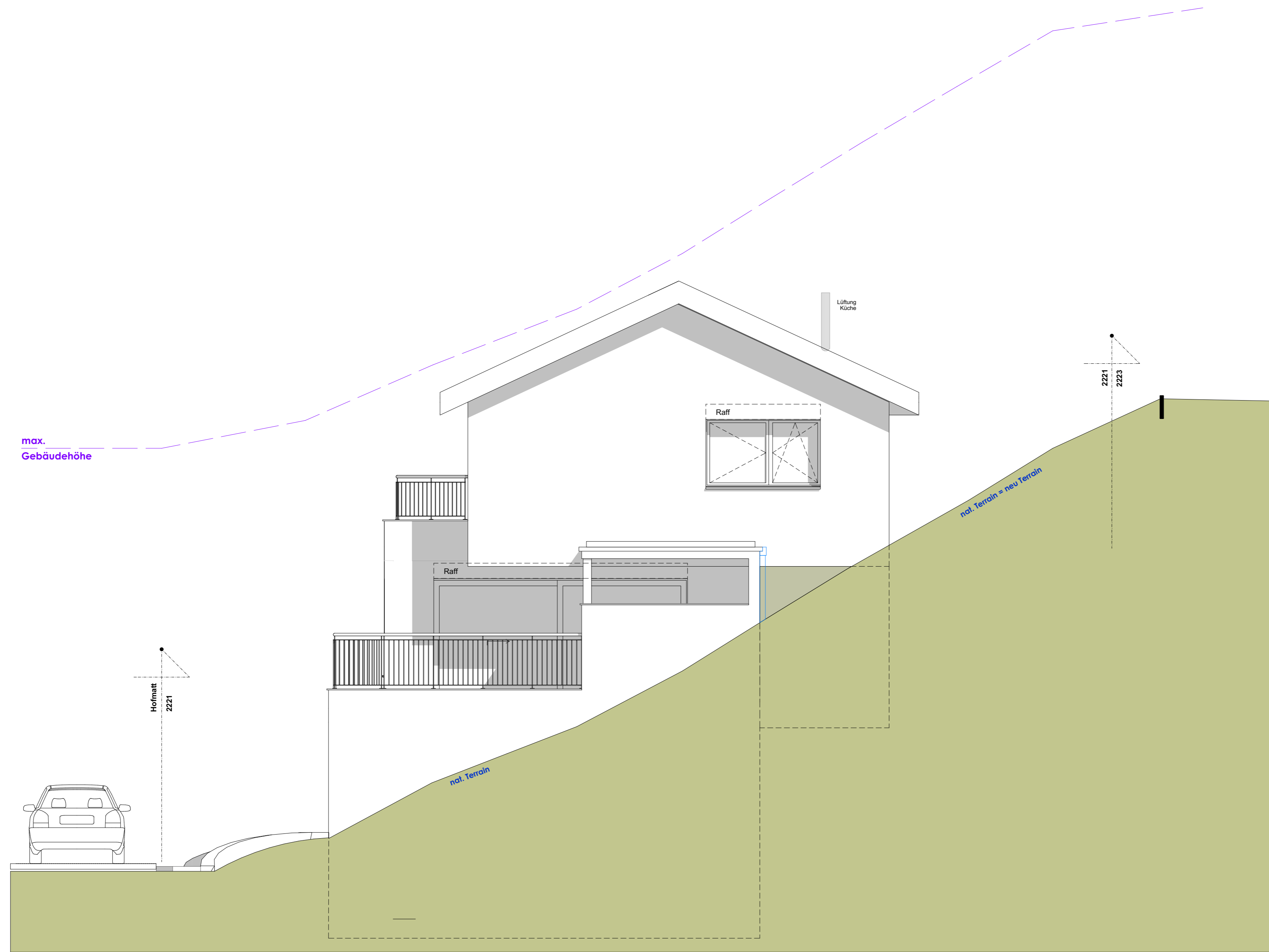
SÜDWESTFASSADE
